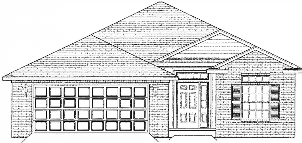
ELEVATION A
